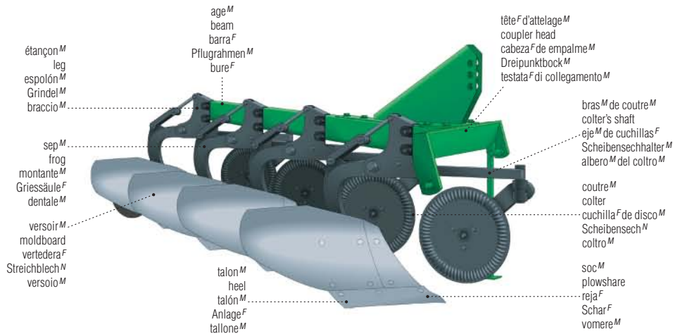
charrue F à soc M ribbing plow arado M de vertedera F Beetpflug M aratro M a vomere M -versoi M
